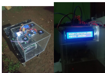
Gambar 3 Tampilan alat
